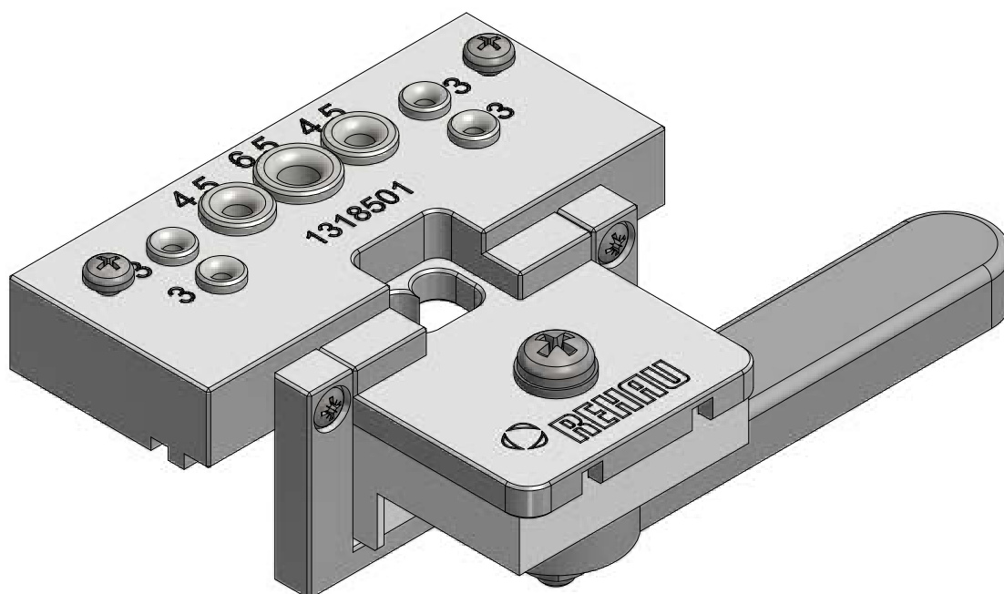
Шаблон для установки мех. соединителей BLITZ New
